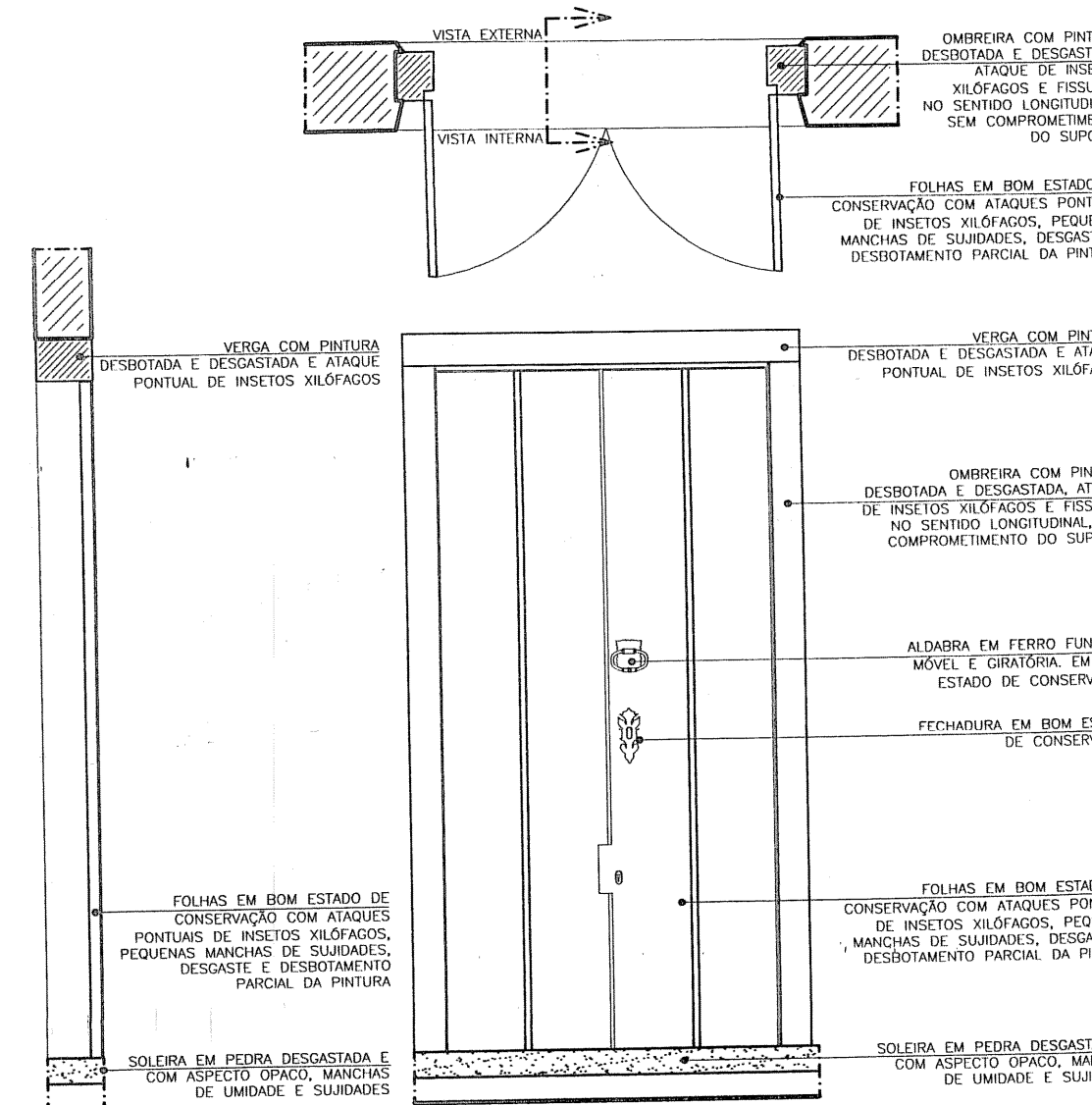
P8 - PLANTA, CORTE E ELEVAÇÕES
