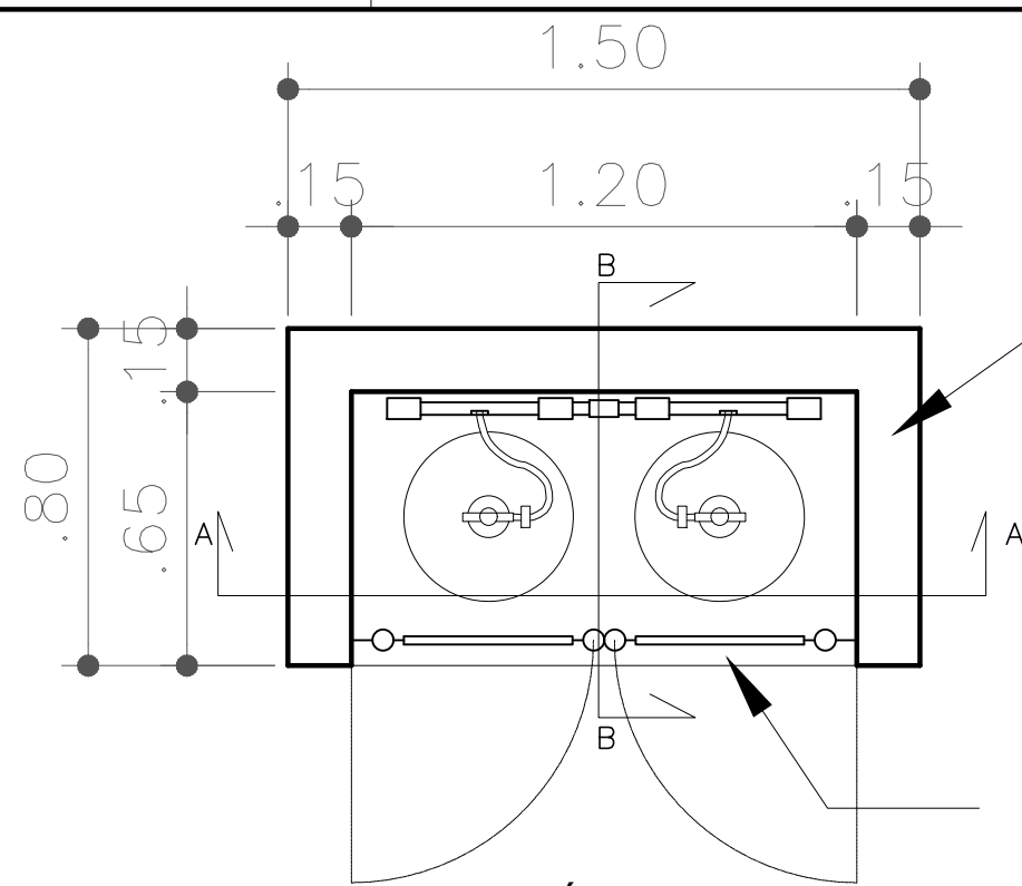
PLANTA BAIXA CENTRAL DE GÁS ESCALA 1/20
