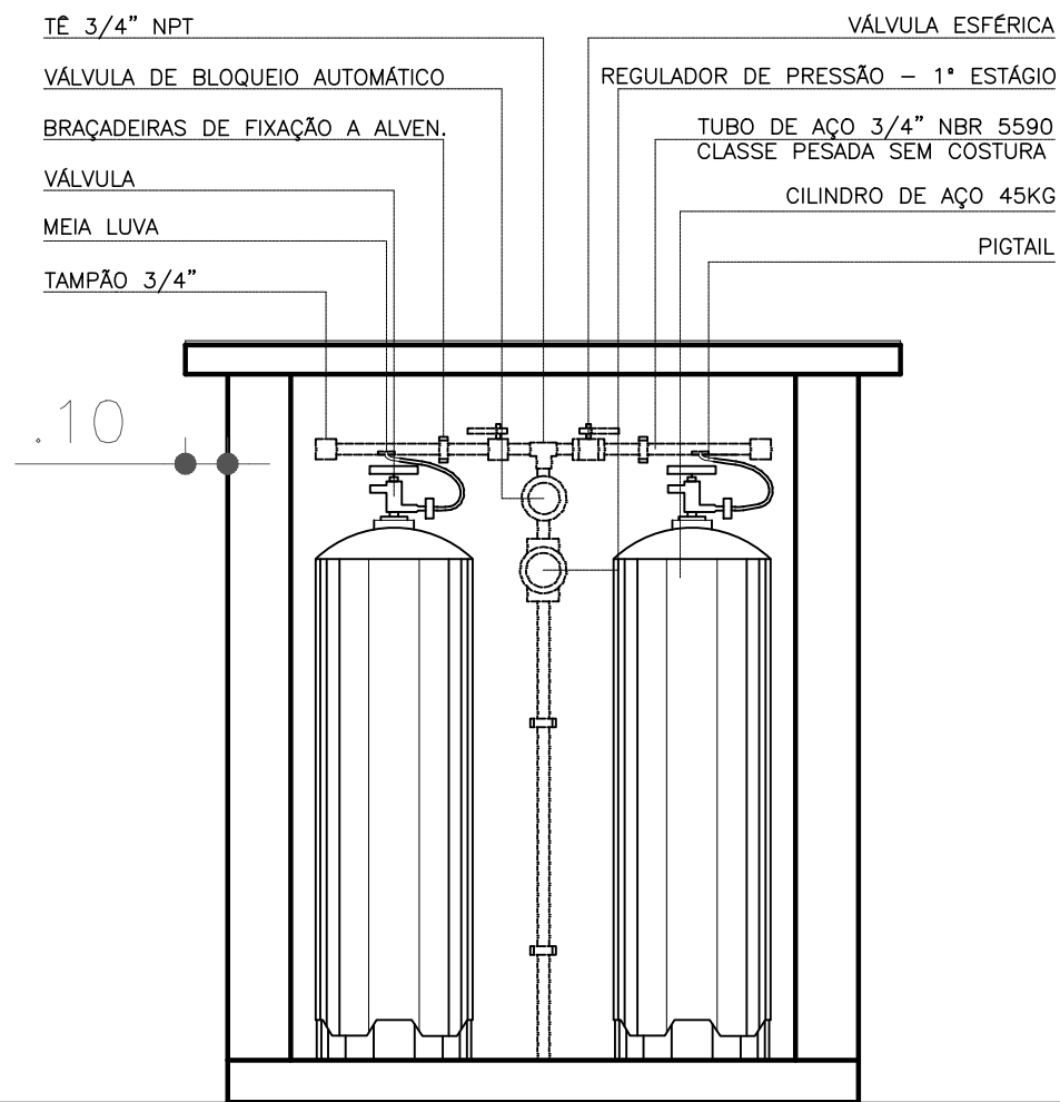
CORTE A'A CENTRAL DE GÁS ESCALA 1/20
