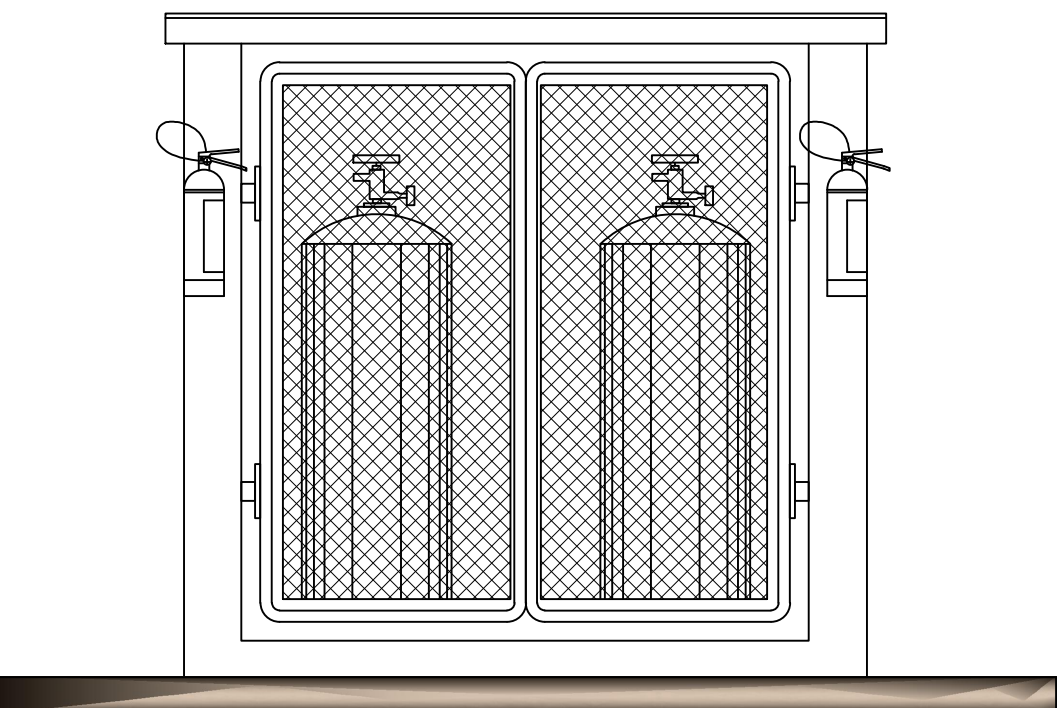
FACHADA CENTRAL DE GÁS ESCALA 1/20
