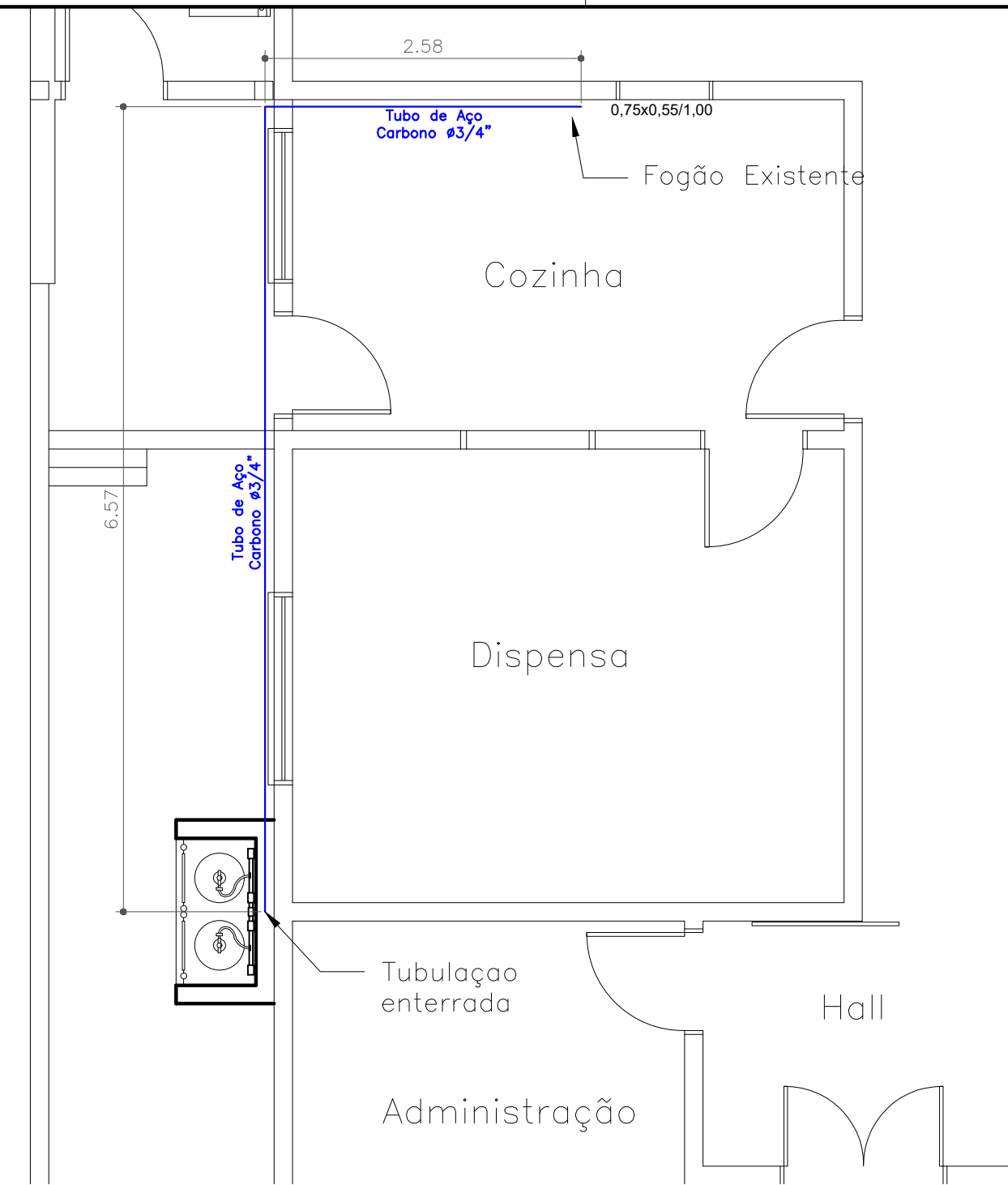
PLANTA BAIXA INSTALAÇÃO DE GÁS ESCALA 1/50
