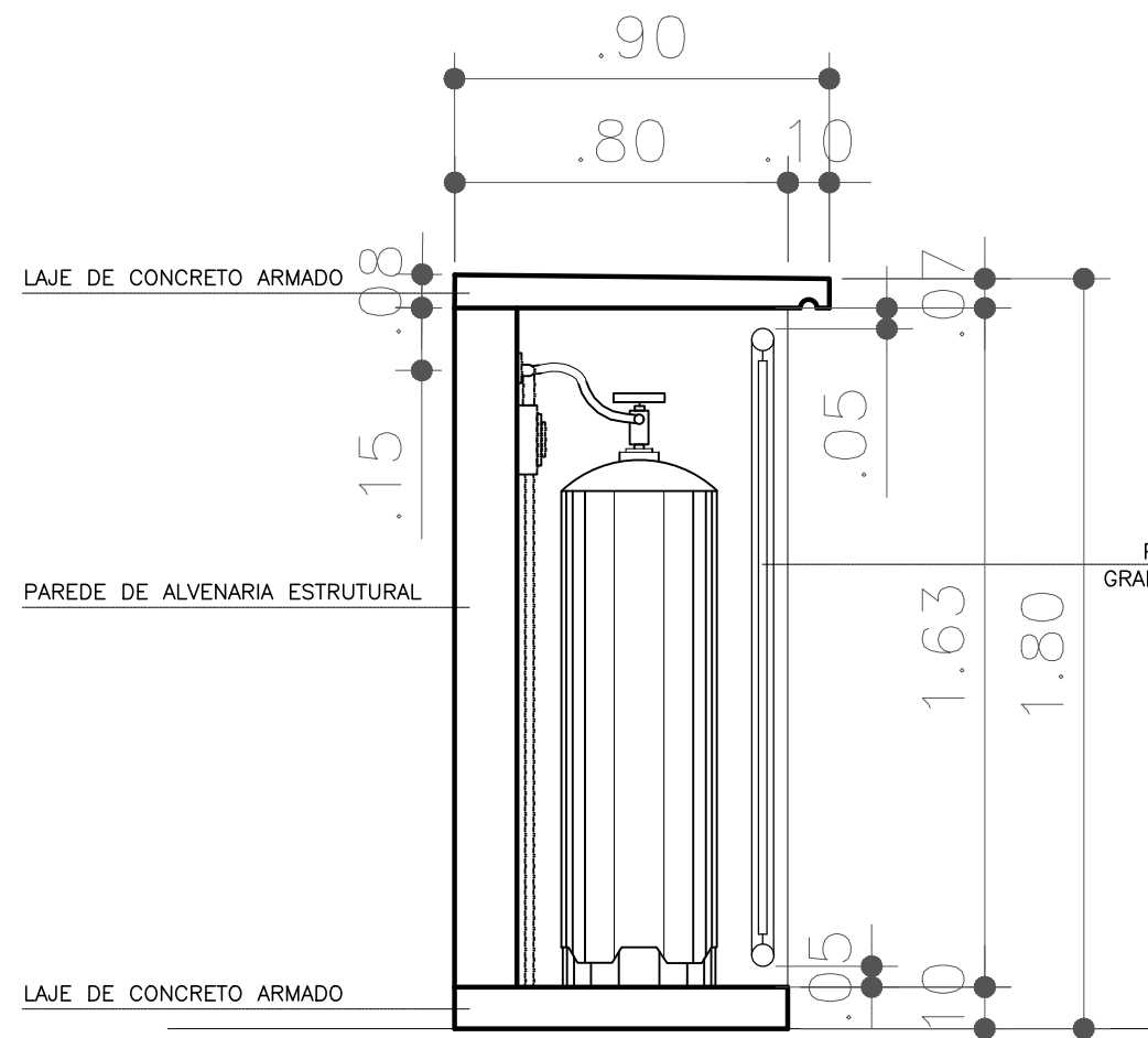
CORTE B'B CENTRAL DE GÁS ESCALA 1/20
