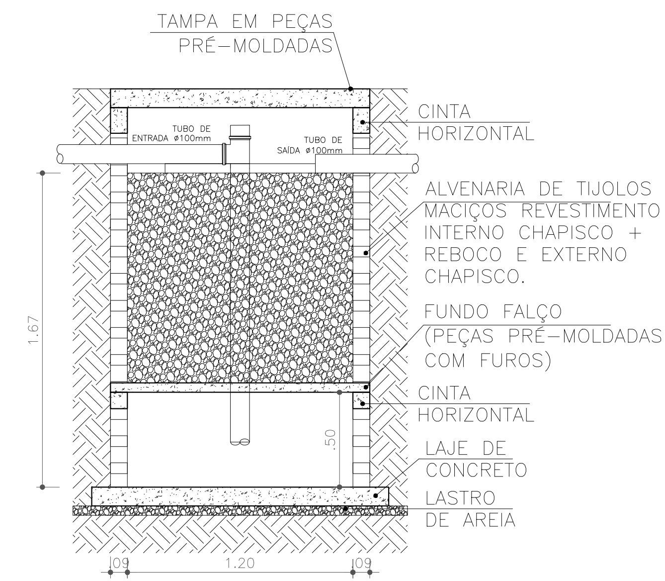
CORTE A/A FILTRO ESCALA 1/20
