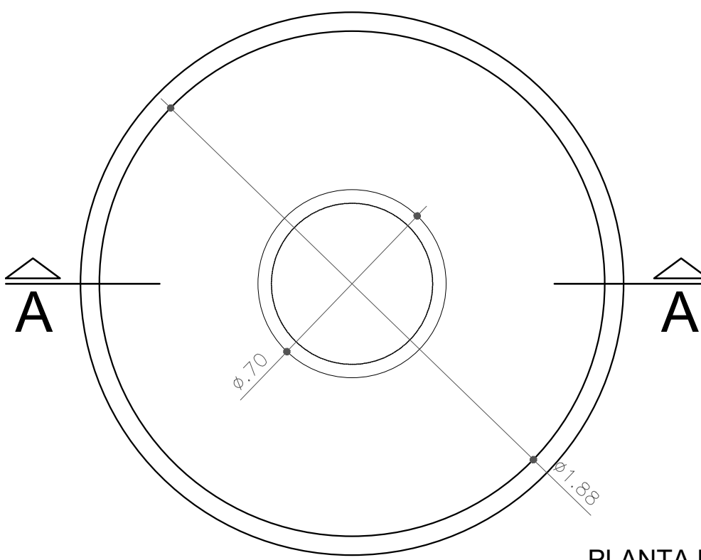
PLANTA BAIXA FOSSA ESCALA 1/20
