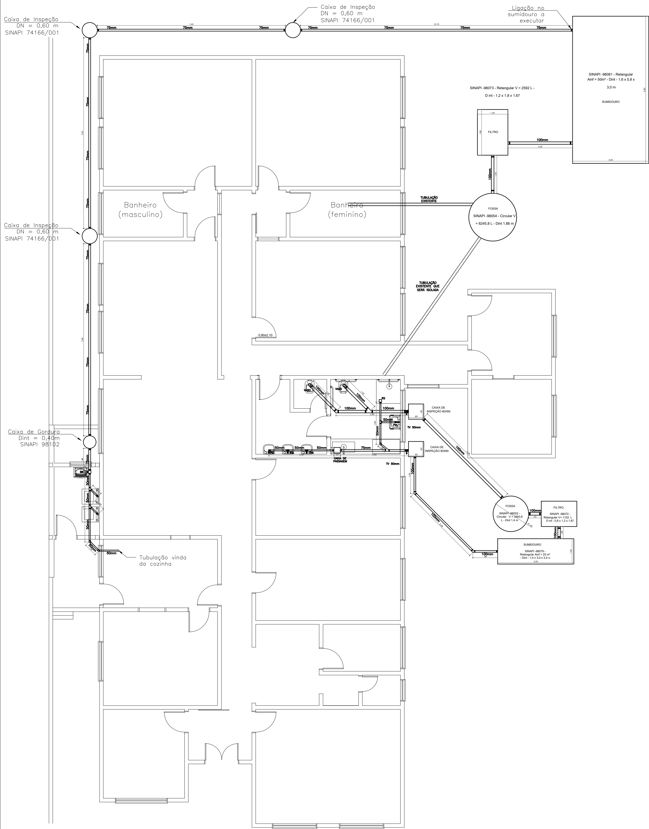
PLANTA BAIXA ESGOTO SANITÁRIO ESCALA 1/75
