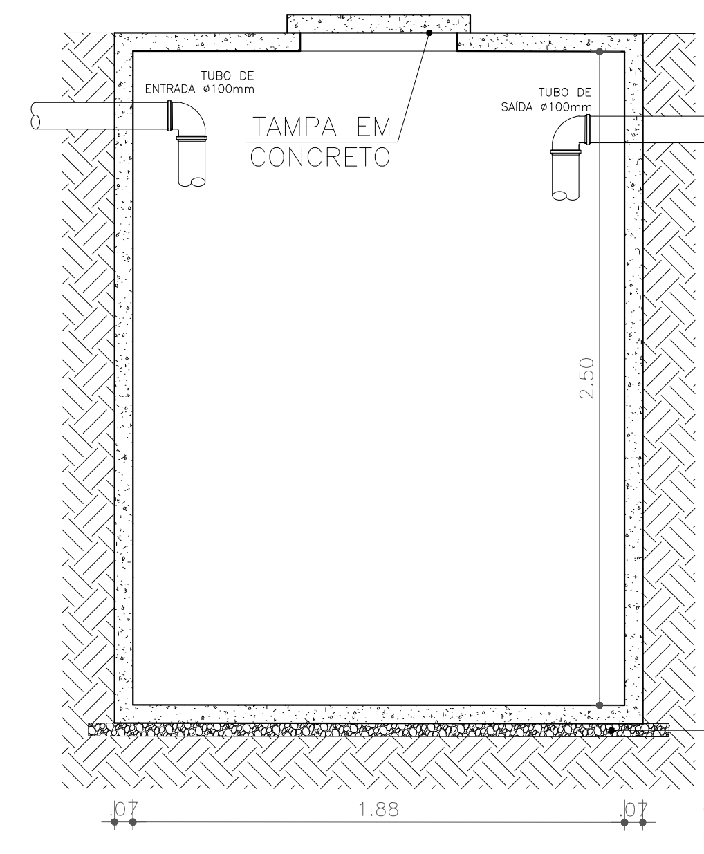
CORTE A/A FOSSA ESCALA 1/20
