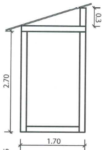
CORTE ESCALA 1/50
