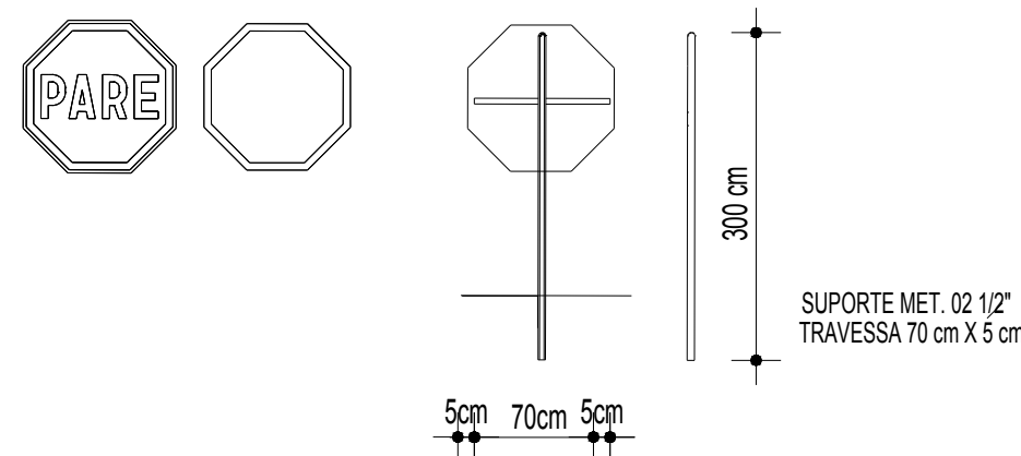
DETALHE PLACAS DE REGULAMENTAÇÃO R-1 FUNDO E ORLA EXTERNA EM VERMELHO, BORDA INTERNA/LETRAS/SÍMBOLOS NA COR BRANCA
