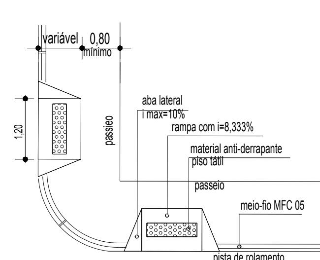
DET. ACESSO PORTAD. DIFICULDADES DE LOCOMOÇÃO S/ESCALA
