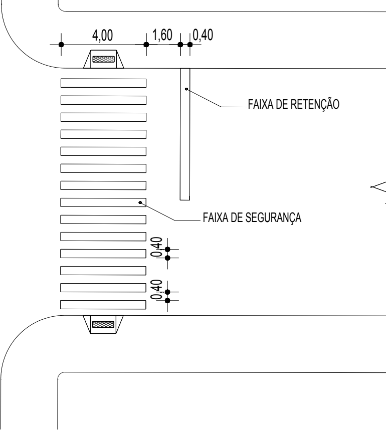
DET. ACESSO PORTAD. DIFICULDADES DE LOCOMOÇÃO S/ESCALA
