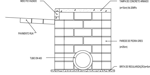
DETALHE SEÇÃO TIPO DA BL S/ESCALA
