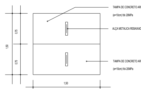
PLANTA BAIXA DA TAMPA S/ESCALA
