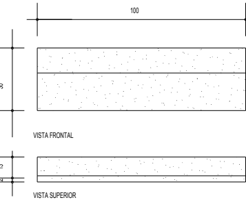
DETALHES DO MEIO FIO S/ESCALA
