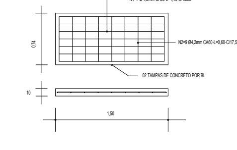
DETALHES DA FERRAGEM DA TAMPA S/ESCALA
