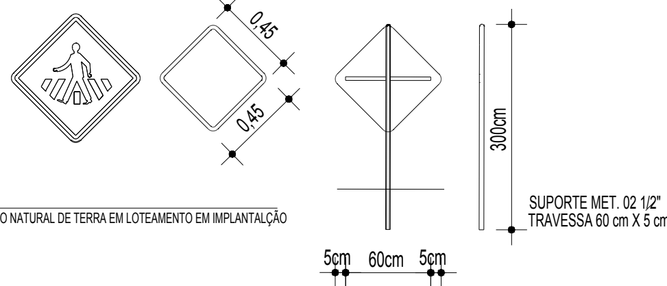
DETALHE PLACAS DE ADVERTÊNCIA A-32B-PASSAGEM SINALIZADA DE PEDESTRES FUNDO E ORLA EXTERNA EM AMARELO, BORDA INTERNA/SÍMBOLOS NA COR PRETA
