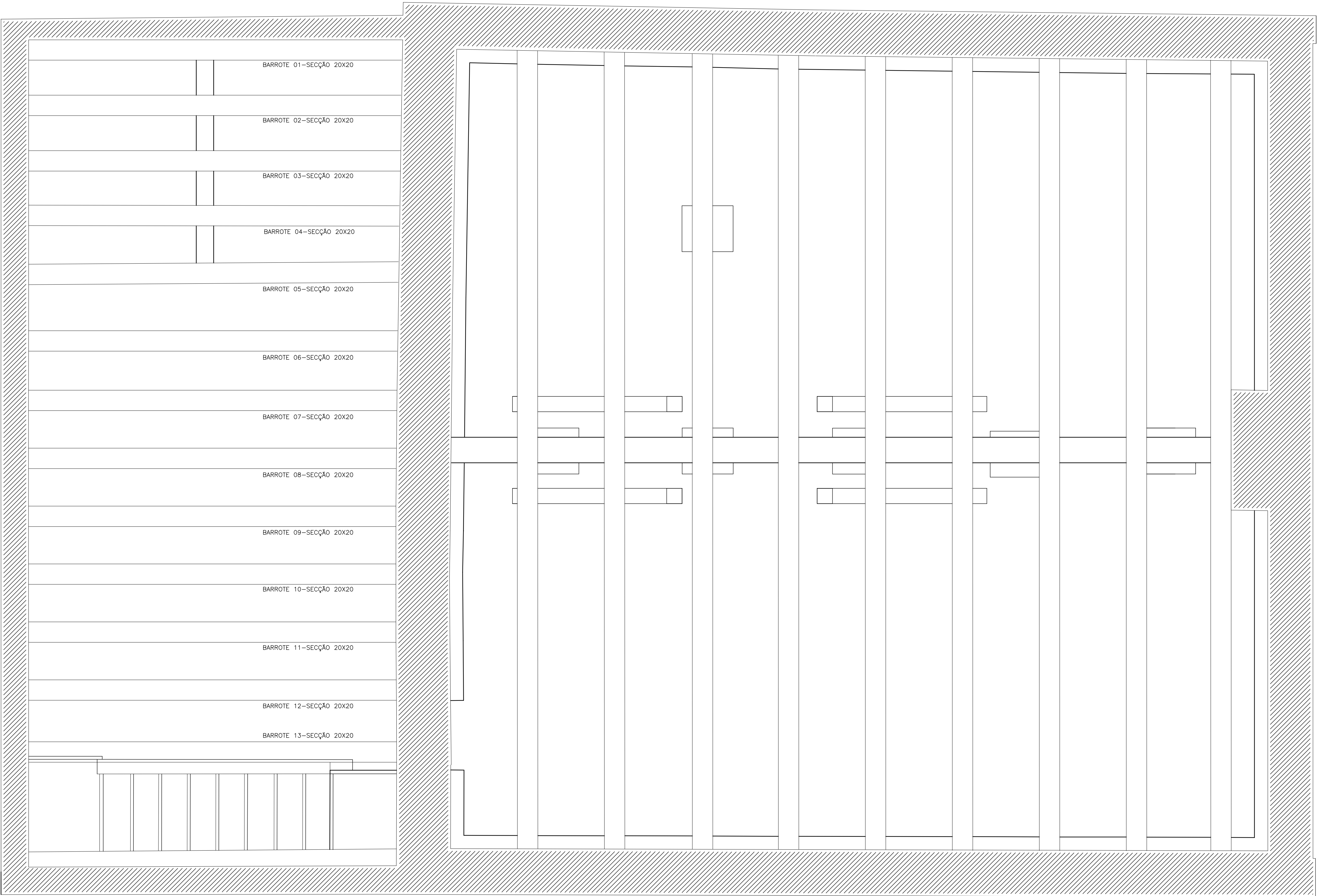
LEVANTAMENTO ARQUITETÔNICO – BARROTES/FORRO – NÍVEL PORÃO
