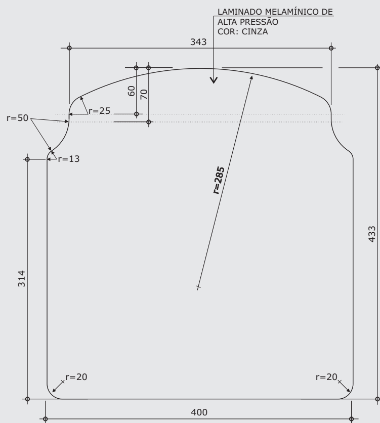
VISTA SUPERIOR
