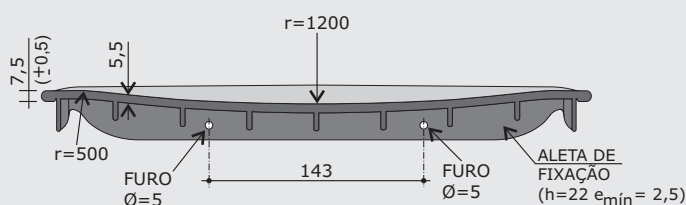
CORTE BB ESC. 1:5
