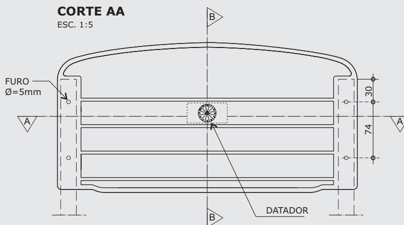
VISTA POSTERIOR
