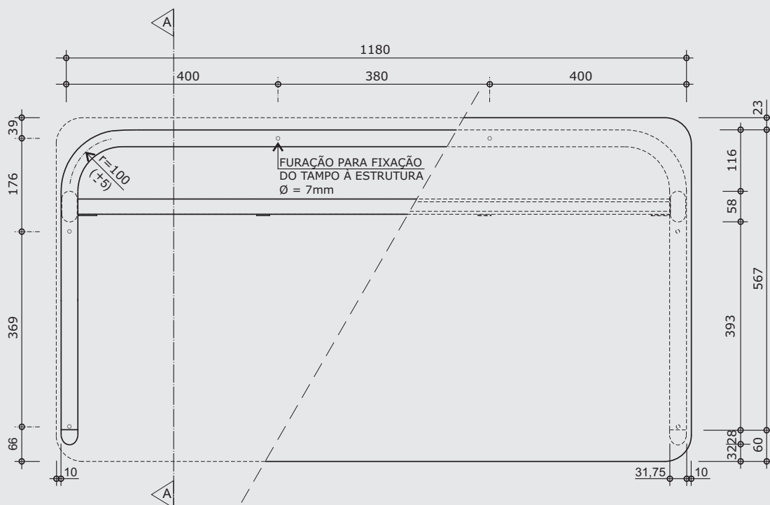
VISTA SUPERIOR
