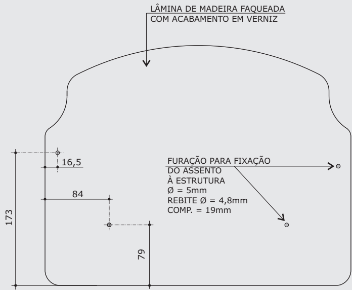
VISTA INFERIOR ESC. 1:5
