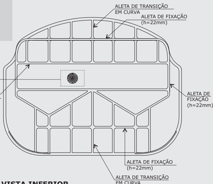
VISTA INFERIOR
