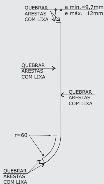
VISTA LATERAL
