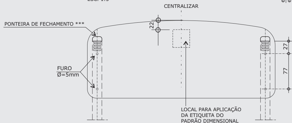
MONTAGEM
