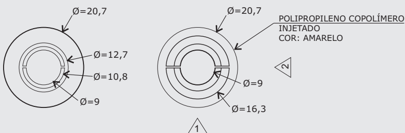
VISTA INFERIOR
