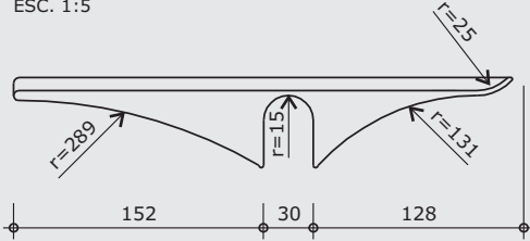
CORTE DD ESC. 1:5
