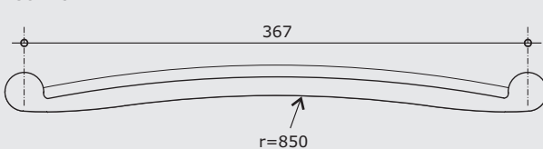
VISTA SUPERIOR
