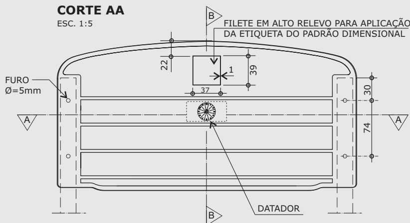
VISTA POSTERIOR
