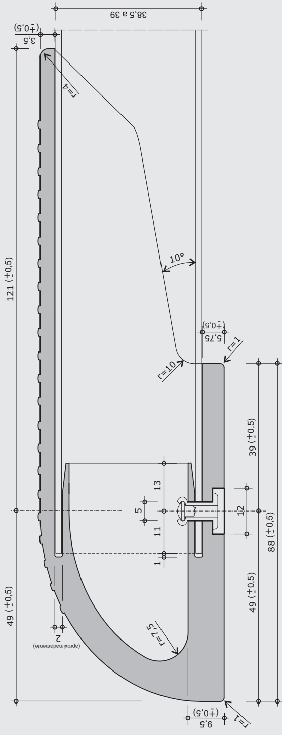
CORTE AA
