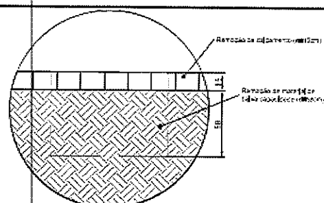
Detalhe de remoção - Áreas de implantação das paradas de ônibus Medidas em centímetros Sem escala Obs: Nas situações em que a área de implantação da parada de ônibus localizar-se sobre uma área de solo de baixa capacidade de suporte, a profundidade de remoção será de 55cm.
