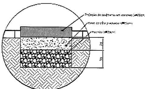
Detalhe de reconstrução do pavimento - Áreas de implantação das paradas de ônibus Medidas em centímetros Sem escala Obs: Nas situações em que a área de implantação da parada de ônibus localizar-se sobre uma área de solo de baixa capacidade de suporte, a profundidade da camada de material para esta situação será de 40cm.
