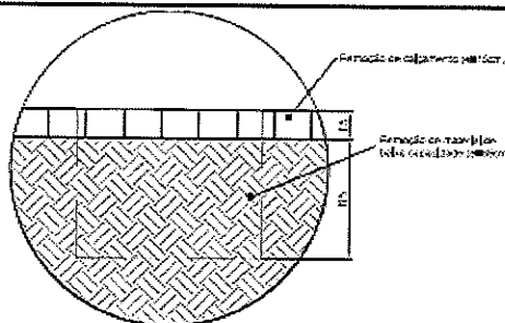
Detalhe de remoção - Área de baixa capacidade de suporte Medidas em centímetros Sem escala
