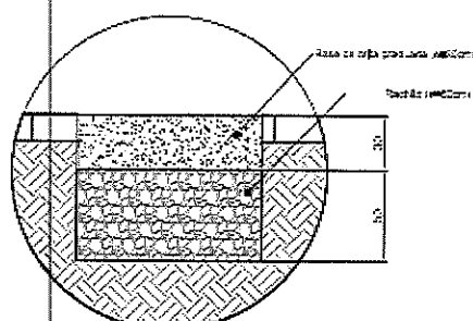
Detalhe de reconstrução do pavimento - Áreas de baixa capacidade de suporte Medidas em centímetros Sem escala
