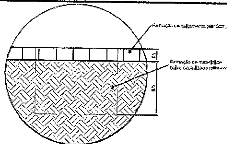
Detalhe de remoção - Áreas de baixa capacidade de suporte Medidas em centímetros Sem escala
