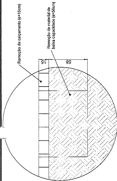
Detalhe de remoção - Áreas de implantação das paradas de ônibus Medidas em centímetros Sem escala
