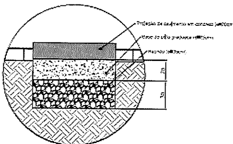
Detalhe de reconstrução do pavimento - Áreas de implantação das paradas de ônibus Medidas em centímetros Sem escala
