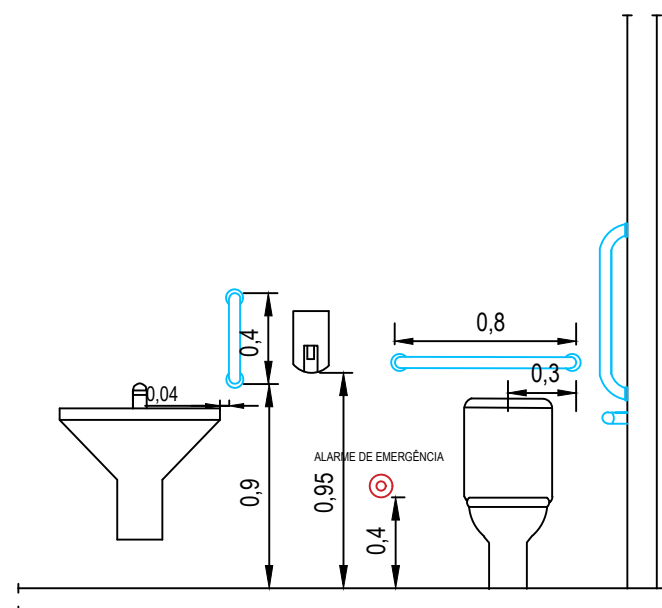
DETALHE BANHEIRO VISTA FRONTAL ESCALA 1:30
