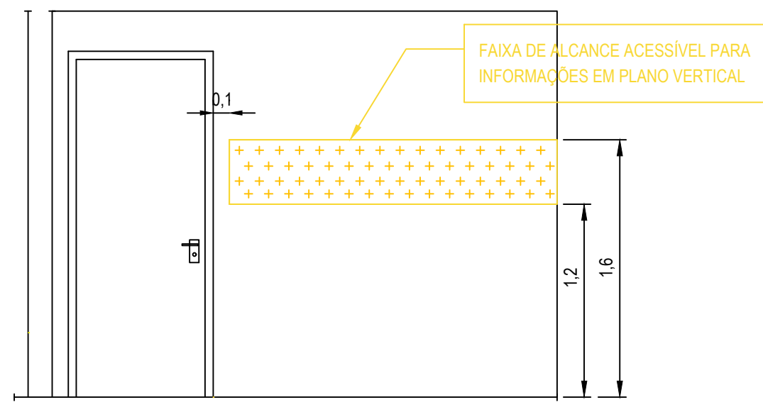
DETALHE SINALIZAÇÃO DE PORTAS VISTA FRONTAL ESCALA 1:30
