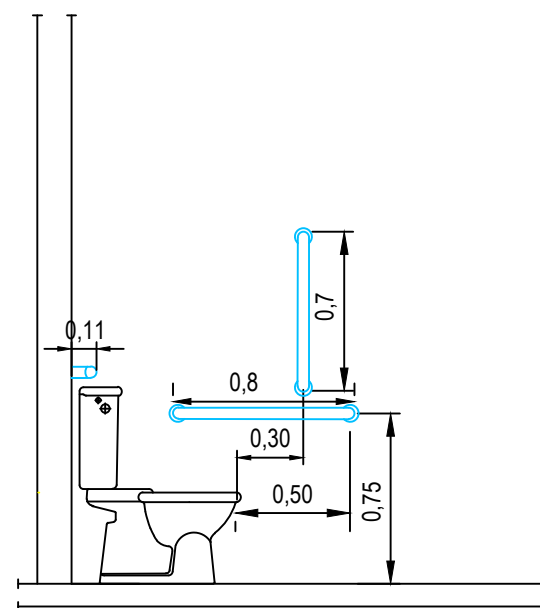
DETALHE BANHEIRO VISTA LATERAL ESCALA 1:30
