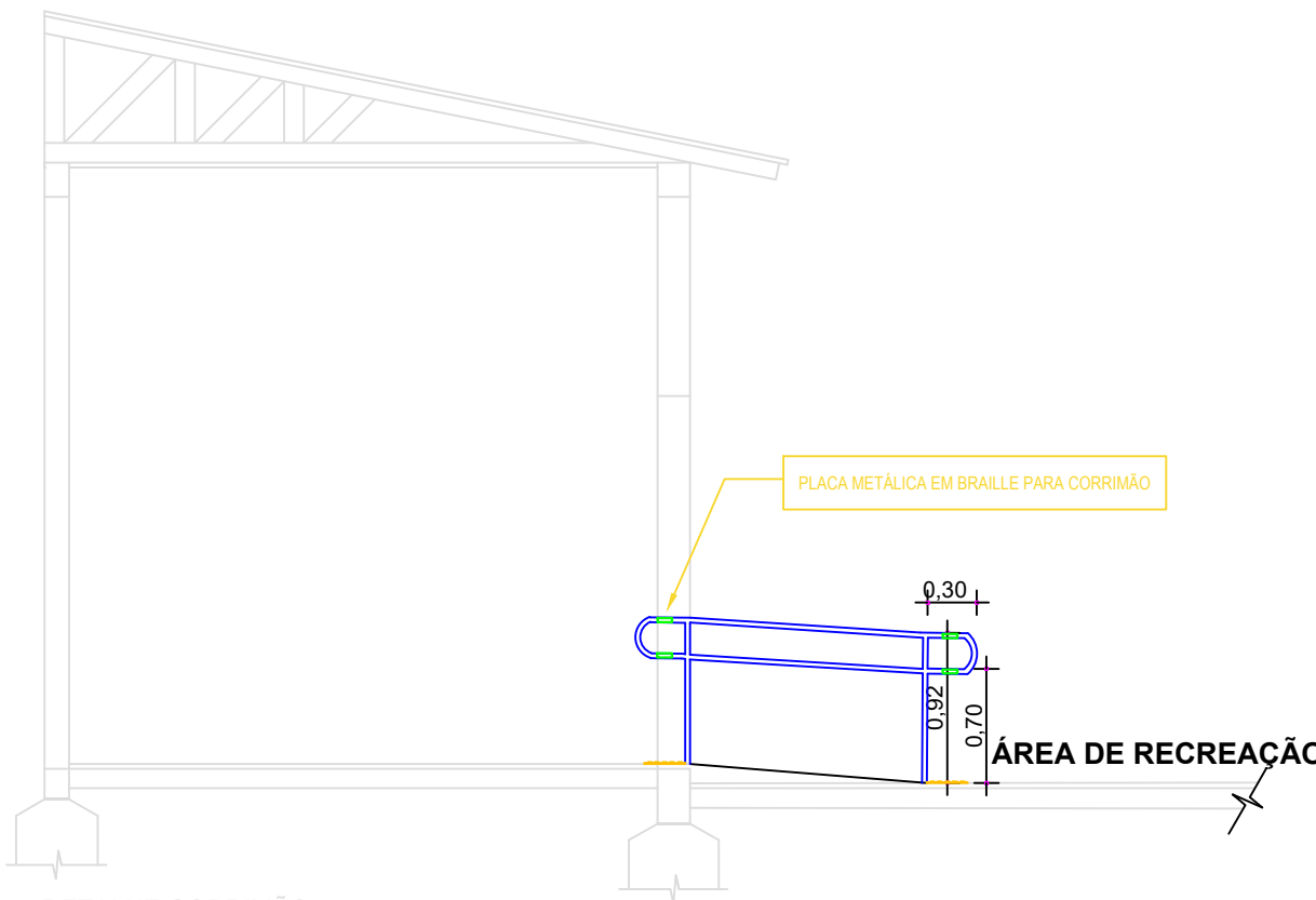
DETALHE CORRIMÃO VISTA LATERAL ESCALA 1:30
