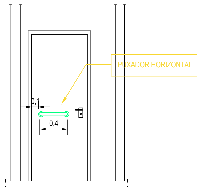
DETALHE BANHEIRO VISTA DA PORTA ESCALA 1:30
