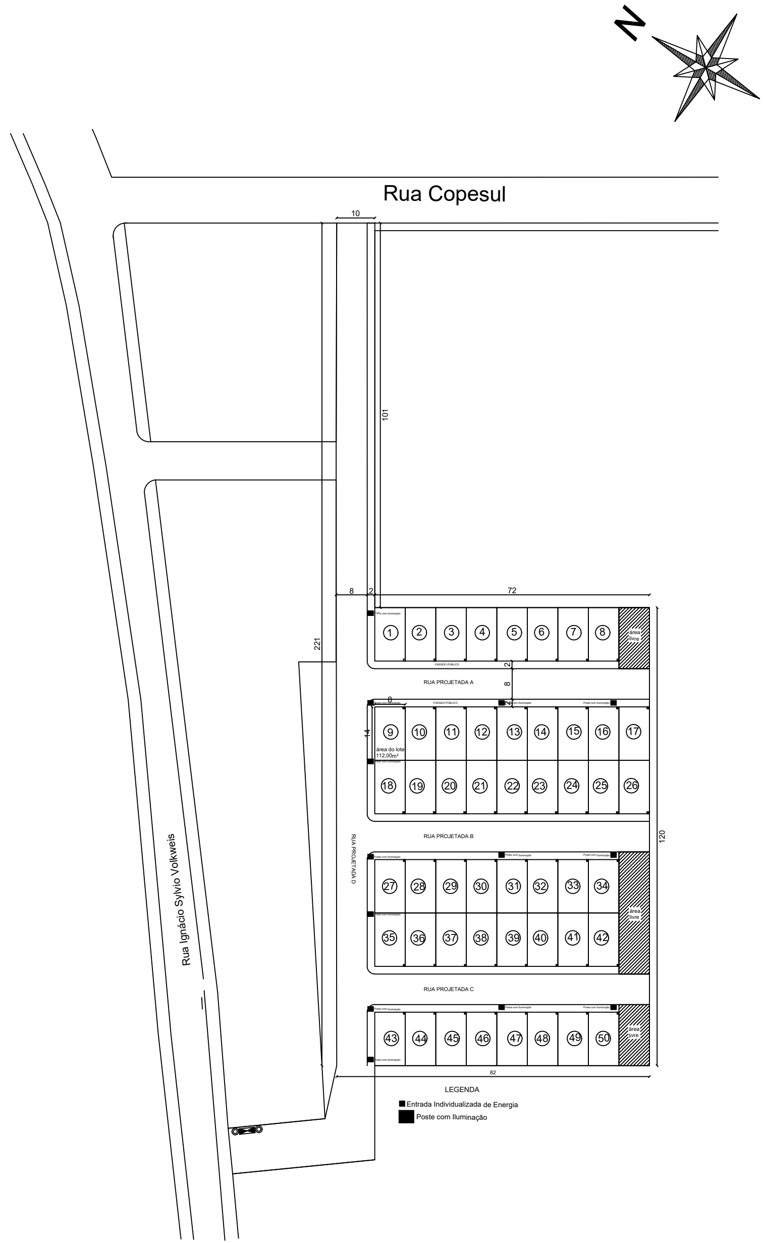
PLANTA DE SITUAÇÃO ESCALA 1/1000
